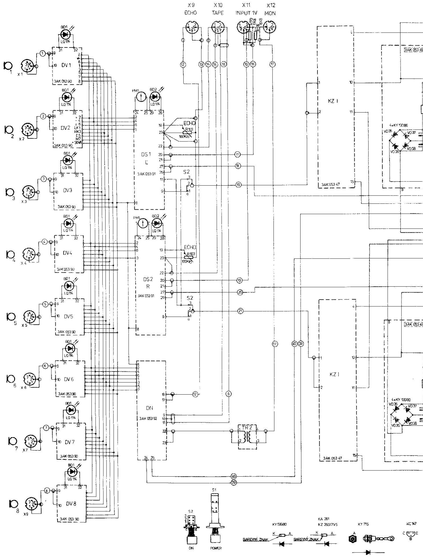
Elektrické blokové schéma
